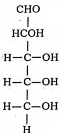
Ribose
