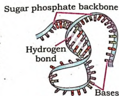
Fig 1.17 rRNA
