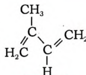
Isoprenoid
