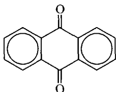
9,10-Anthraquinone
