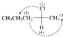
( S )-2-Chloropentane
